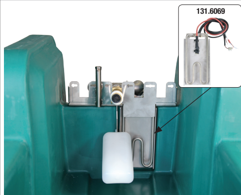
Нагревательный тэн
