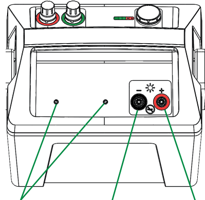
Orifices de montage pour le support Raccordement solaire (-) Raccordement solaire (+)
