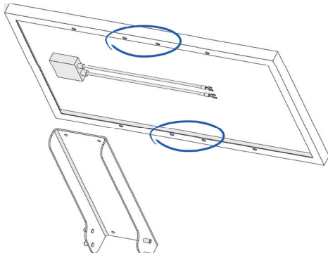
Module solaire 20 W / 40 W
