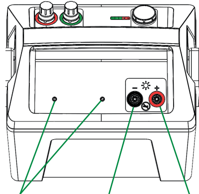
Montagegaten voor zonnepaneel houder Zonne-energie aansluiting (-) Zonne-energie aansluiting (+)
