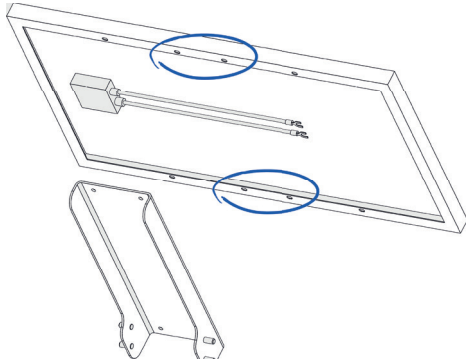
Módulo solar 20 W / 40 W
