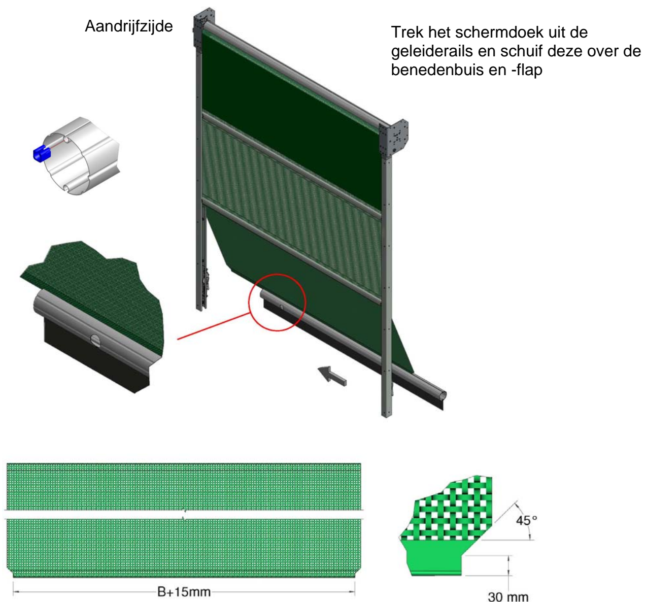
Afbeelding 14b, Bevestigen van benedenbuis
