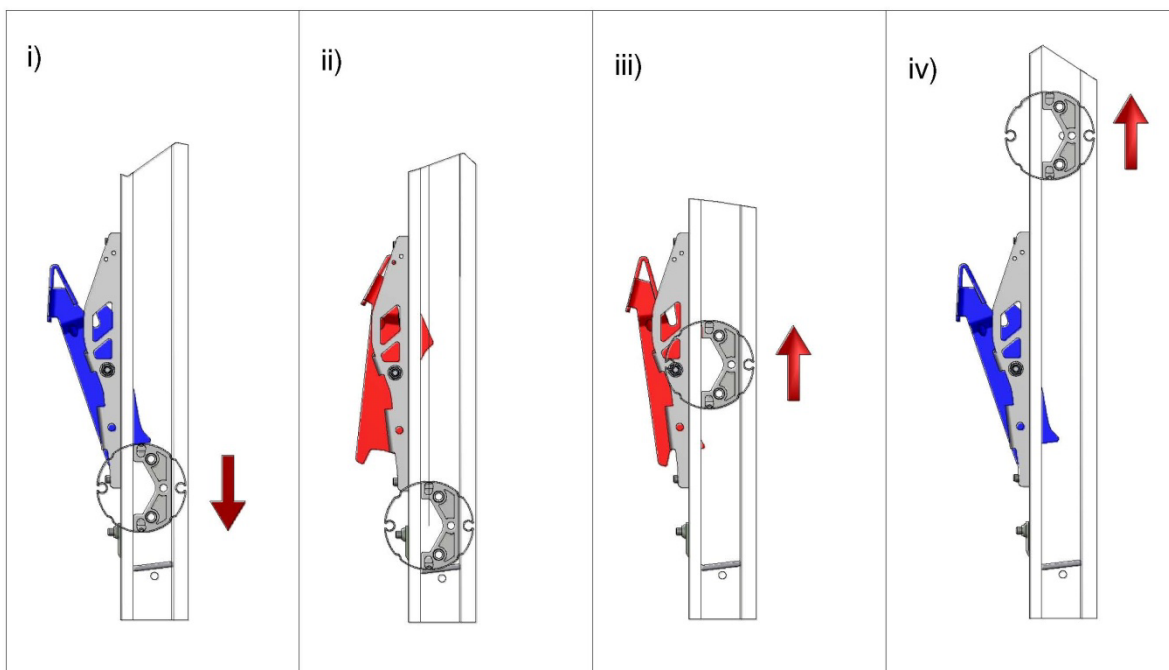
Afbeelding 25, Deur openen
