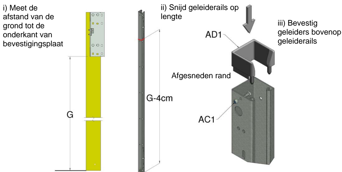
Afbeelding 10, Geleiderails op maat snijden
