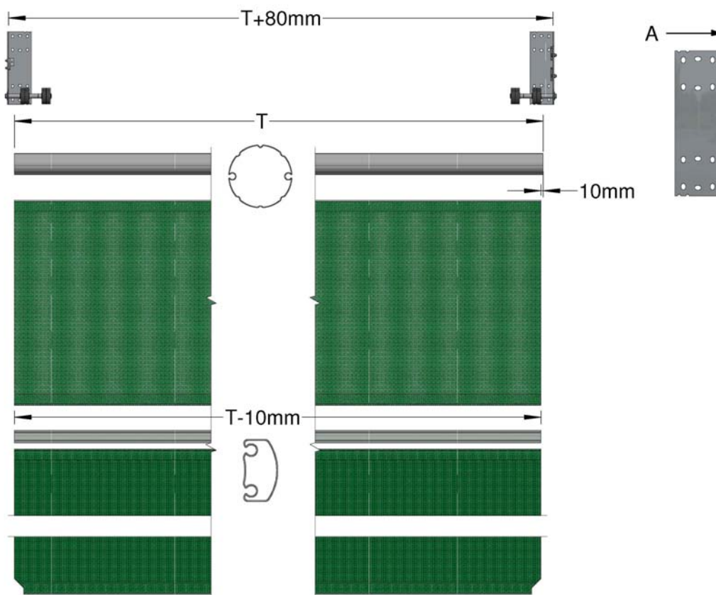
Afbeelding 4b, Tussenruimte voor bovenste bevestigingsplaat wanneer buis, windijzers en ventilatiedoek niet op maat worden gesneden
