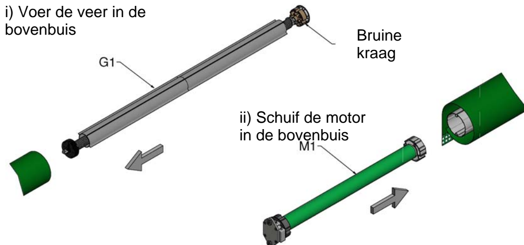
Afbeelding 6b, Bovenbuismontage (rechtse aandrijving)
