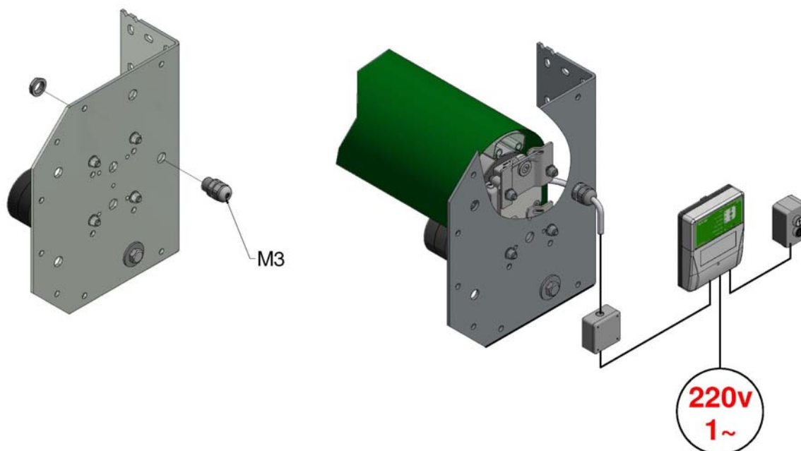
Afbeelding 8a, Aanbrengen van motorbedrading
