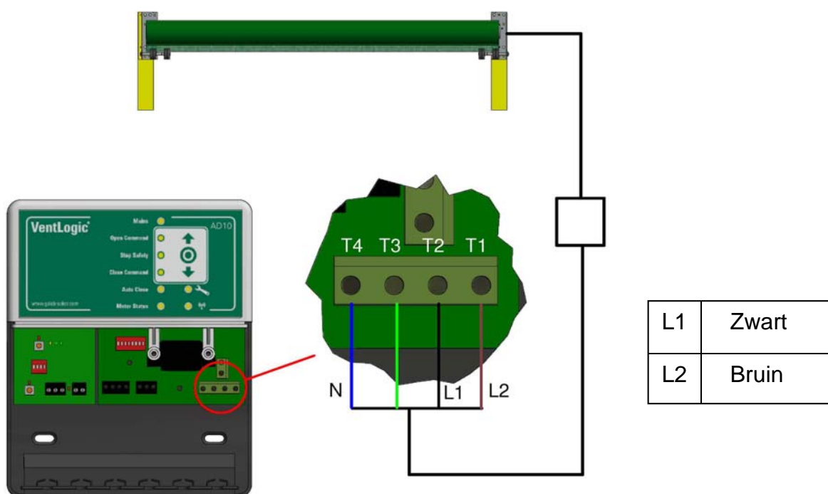
Figuur 8b, Bedrading van bedieningskast
