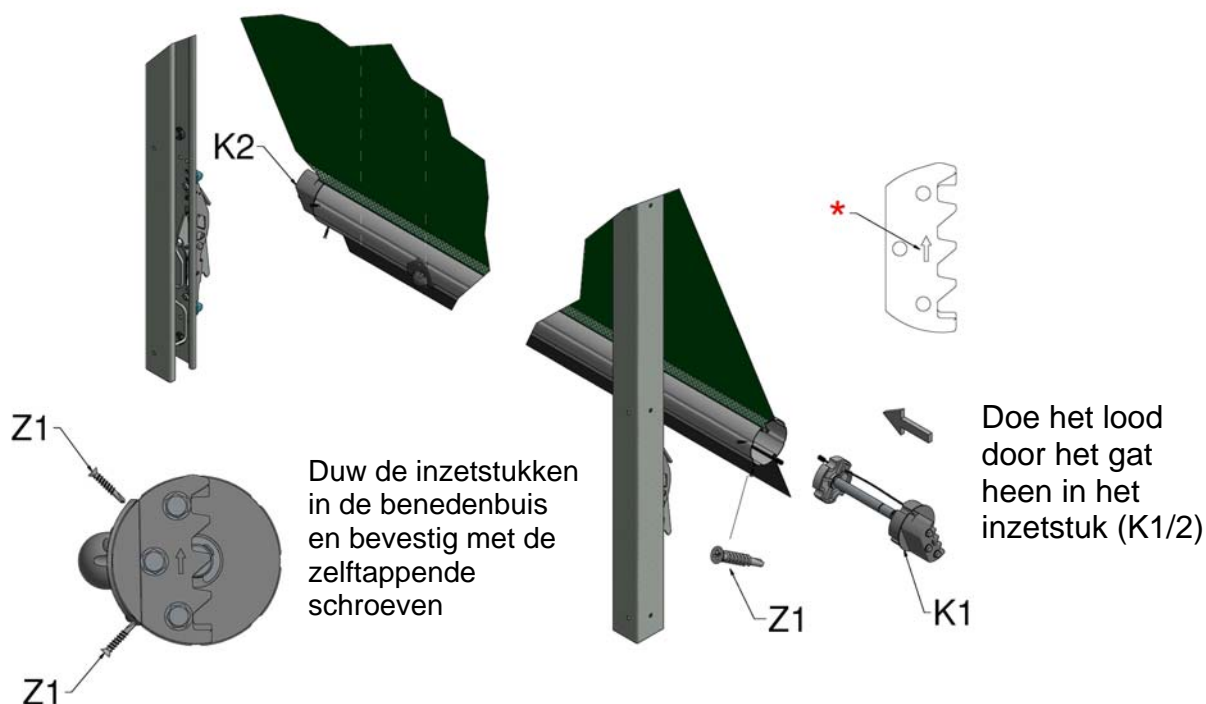
Afbeelding 15b, Inzetstuk benedenbuis
