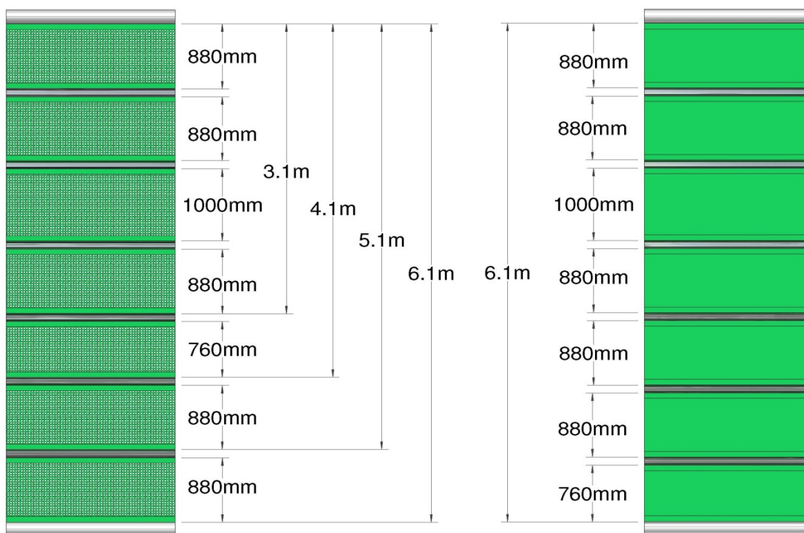
Afbeelding 5b, Ventilatiepaneel-layout
