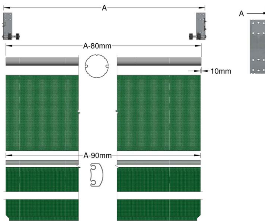
Afbeelding 4a, Op lengte snijden van buizen en doek
