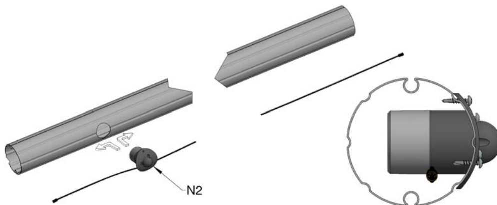
Afbeelding 15a, Monteer de Zender in benedenbuis
