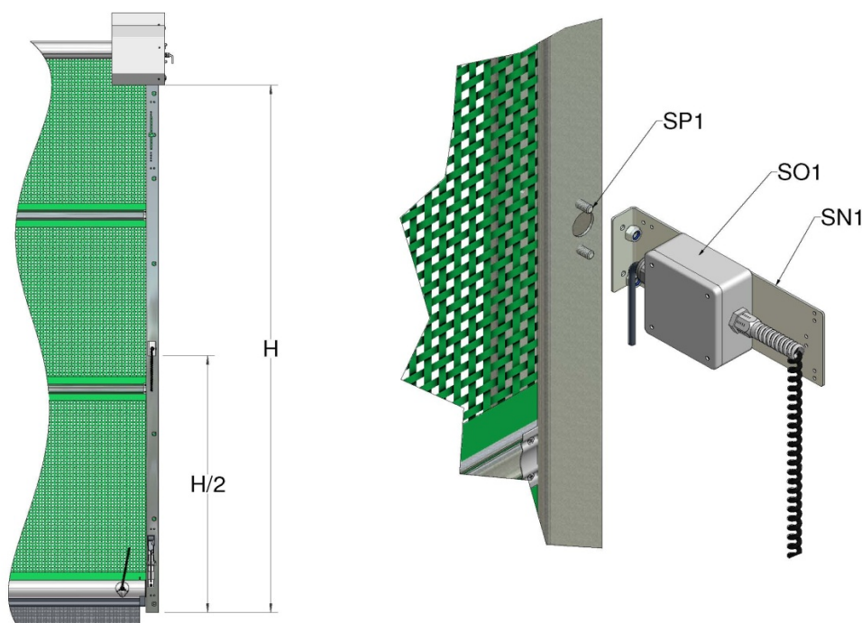
Afbeelding 29, Verloopsteun
