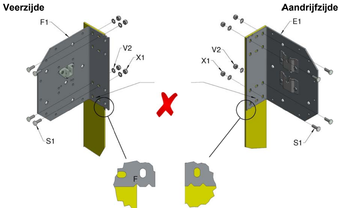
Afbeelding 3, Plaatsing van de bovenste bevestigingsplaat
