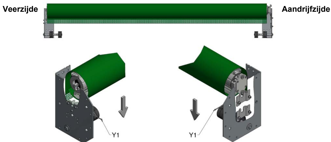
Afbeelding 7, Bovenbuis in bevestigingen plaatsen (rechtse aandrijving getoond)
