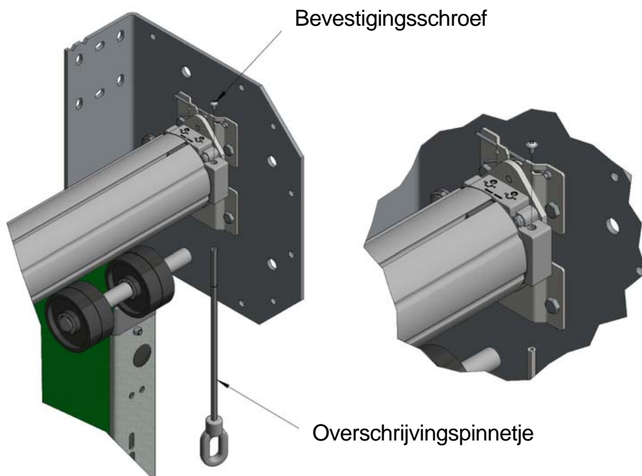
Figuur 19, handmatig overschrijvingspinnetje
