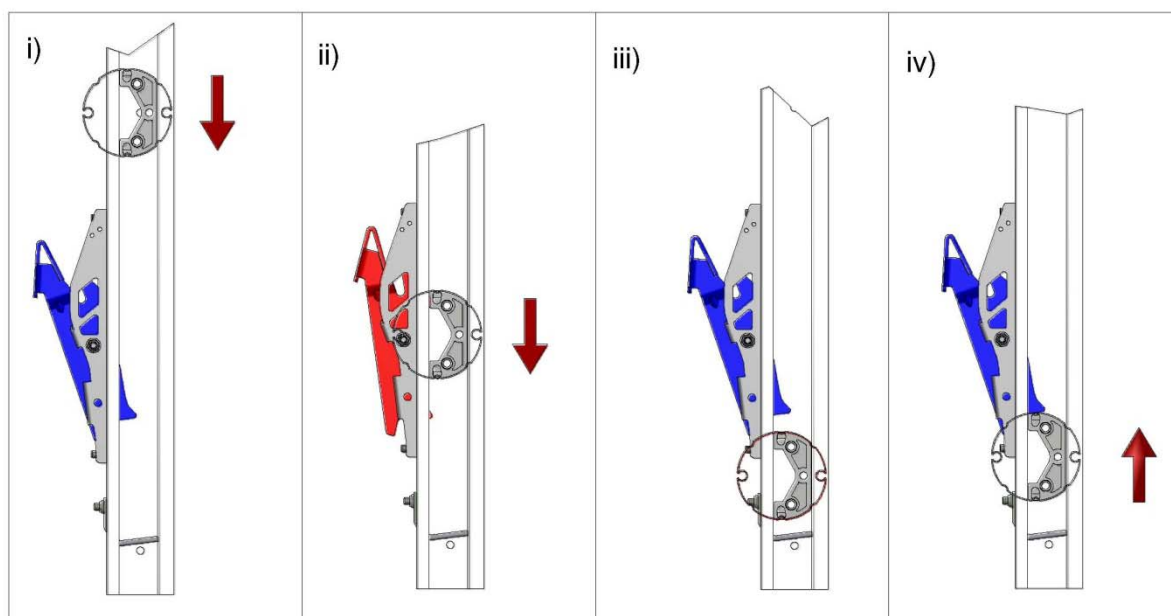
Afbeelding 24, Deur sluiten
