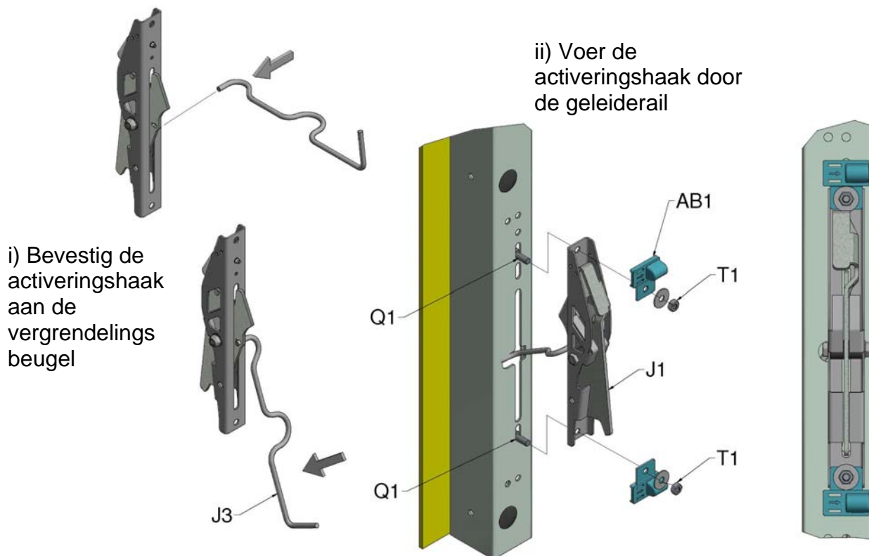
Afbeelding 12, Bevestiging van vergrendelingspallen
