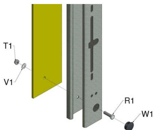
Afbeelding 11b, Bevestiging van geleiderail aan de muur
