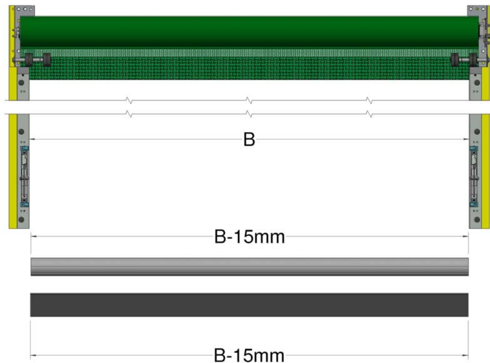
Afbeelding 14a, Op lengte snijden van benedenbuis en benedenflap
