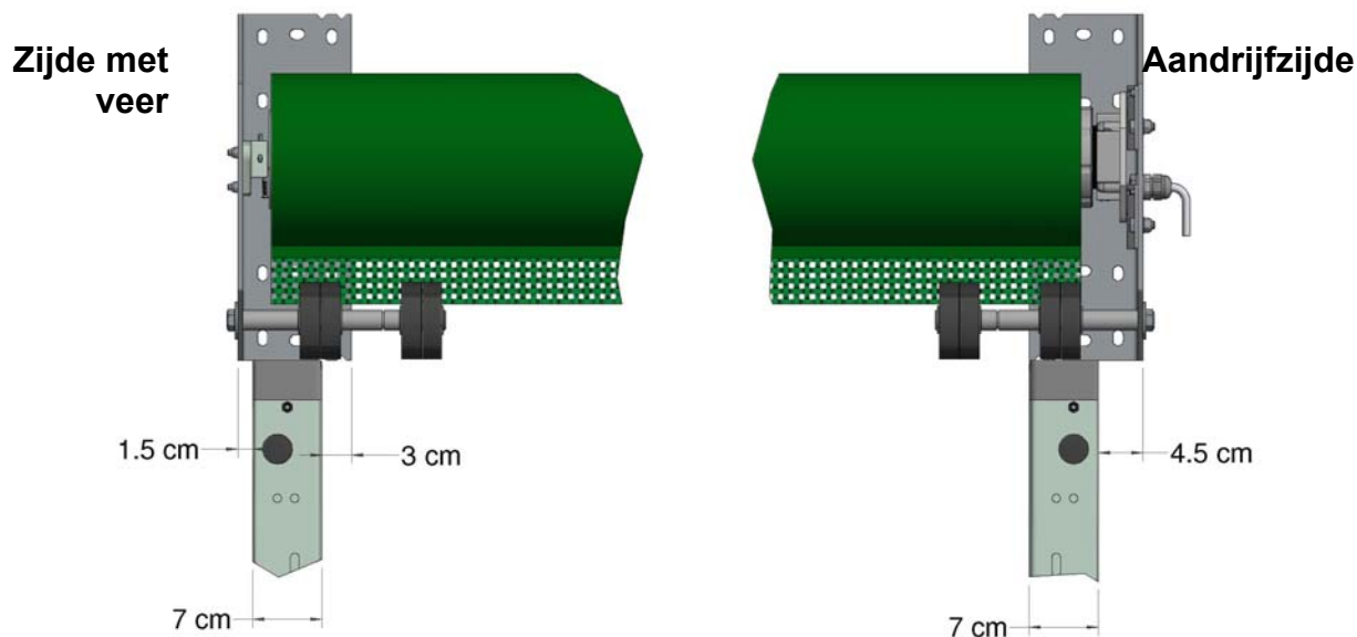
Afbeelding 11a, Plaatsing van de geleiderails
