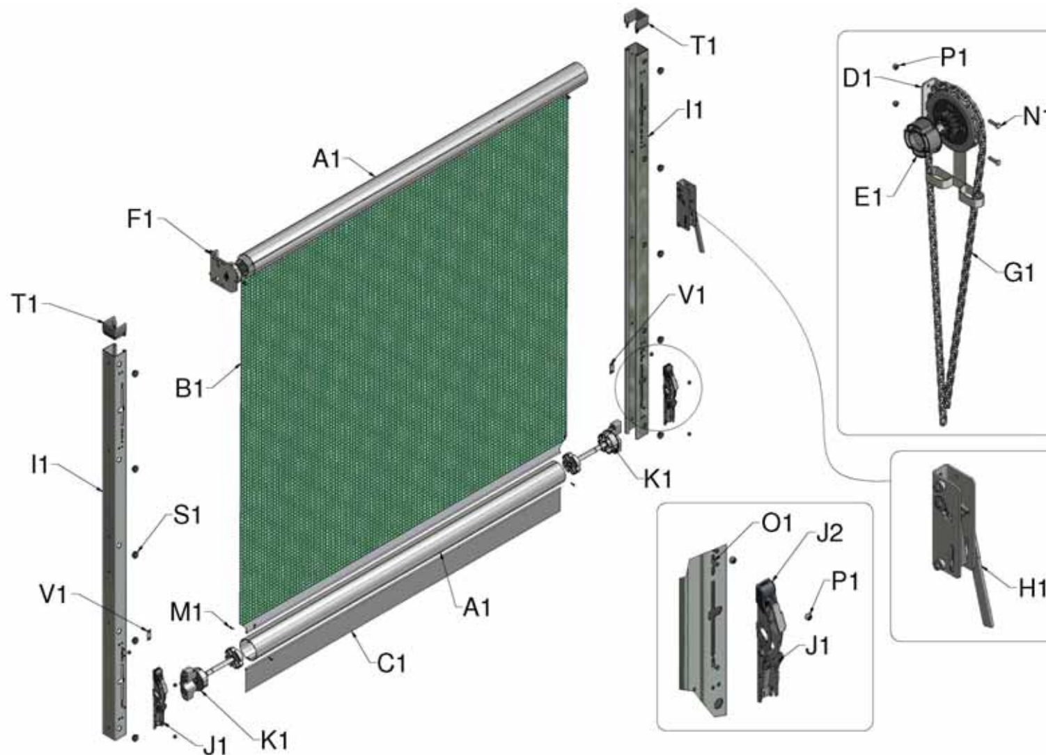
Afbeelding 1, Systeemoverzicht en de onderdelen apart
