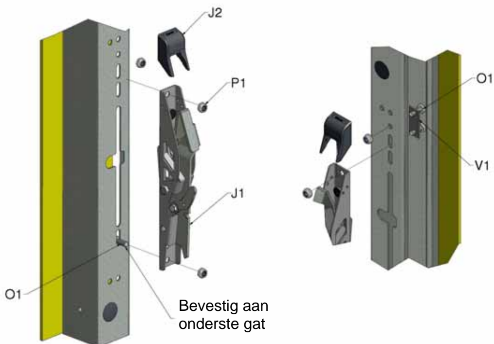
Afbeelding 9, Bevestiging van geleiderails
