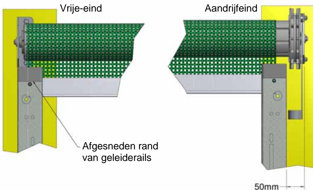
Afbeelding 8a, Plaatsing van de geleiderails
